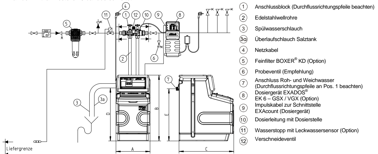
Abb. 2: Aufstellungszeichnung WINNI-mat® VGX
